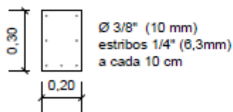
5 DET. CINTAS ESCALA: 1/25
