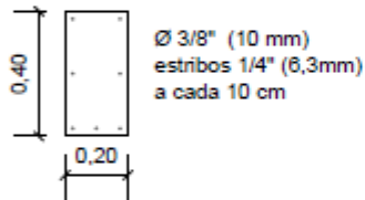
4 DET. VIGA BALDRAME ESCALA: 1/25
