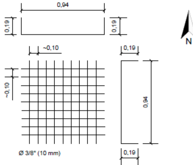
3 DET. ARMAÇÃO DAS SAPATAS ESCALA: 1/25
